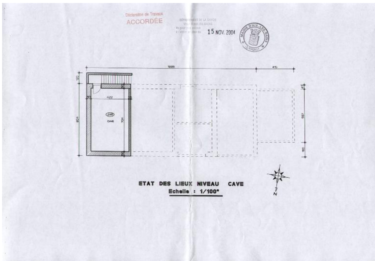
Plan du sous-sol avant travaux, 2004
