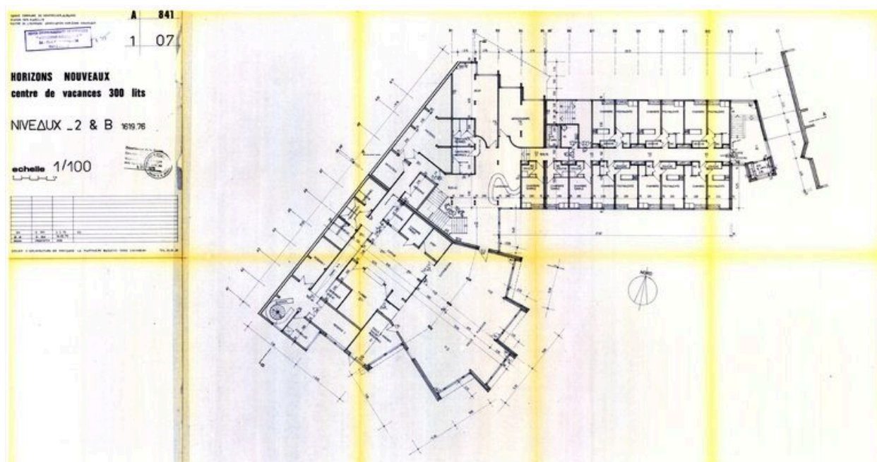
Horizons nouveaux. Centre de vacances 300 Lits. Plan niveaux -2 et B / Atelier d'architecture en Montagne, Guy Rey-Millet, 14 février 1975 (AC Montricher-Albanne)
