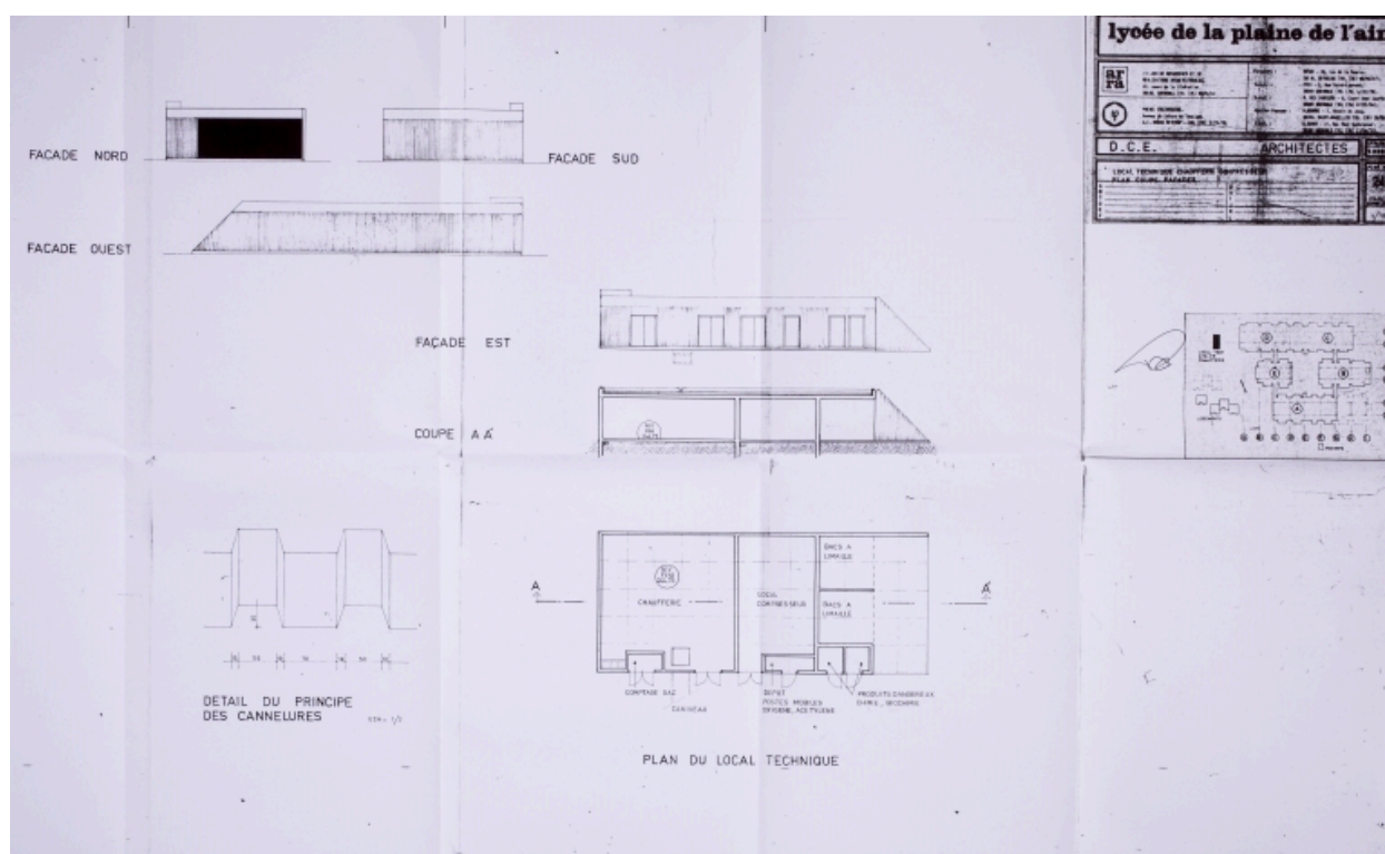
D.C.E. Equipements solaires. Plan du local technique, détail du principe des cannelures. 31 mars 1981. ARRA, Phénol Engineering. Document figuré. Papier. 1/100e. 1981. Archives du lycée de la Plaine de l'Ain, Ambérieu-en-Bugey. non coté
