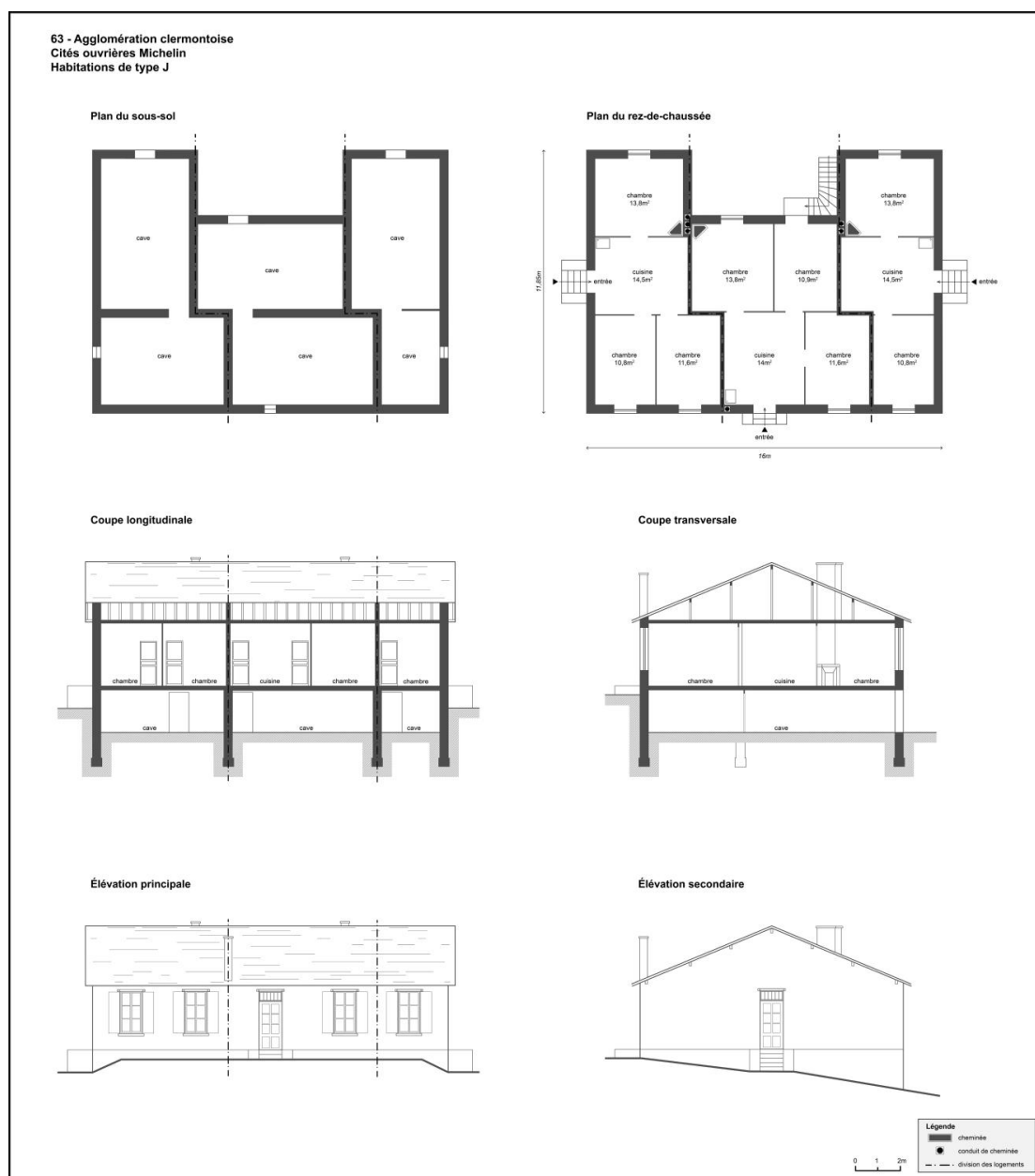
Plans, coupes, façades des habitations de type J
