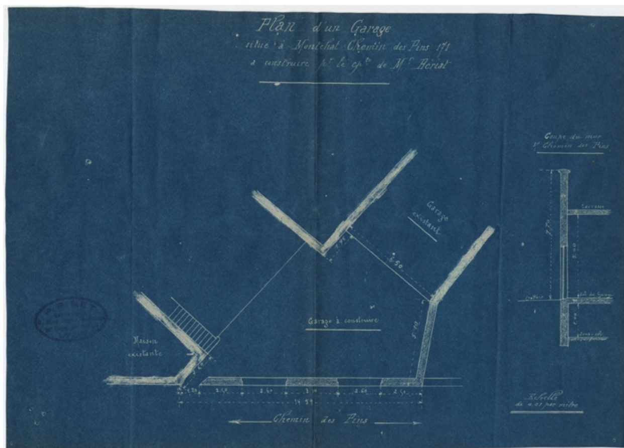
AC Lyon : 344 WP 217 PCA n° 0760, plan du garage pour M.Bériat par M. Pinet, 1926
