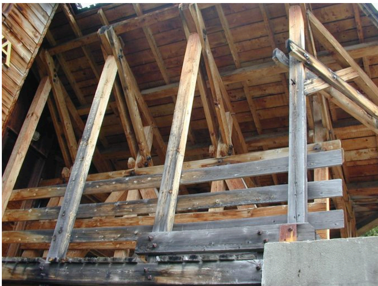
La charpente de la galerie d'entrée
