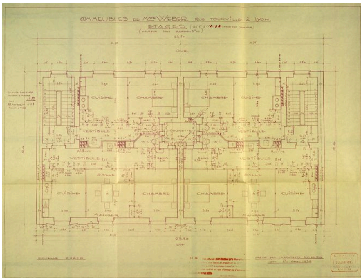
Plan des étages / L. Gandy architecte, 20 septembre 1935 (AC Lyon. 1097WP 577)
