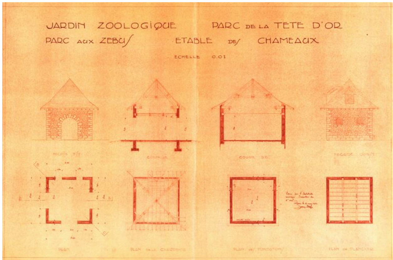
Parc aux zébus, étable des chameaux, plans, coupes, élévations, Jean Dorel, 1953
