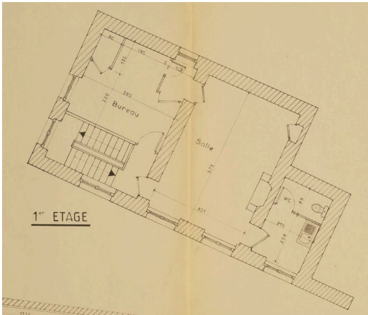
Détail du plan de l'immeuble Montalembert, 1er étage, L. Brassart, 1992 (AP Lycée Saint-Paul Forez).
