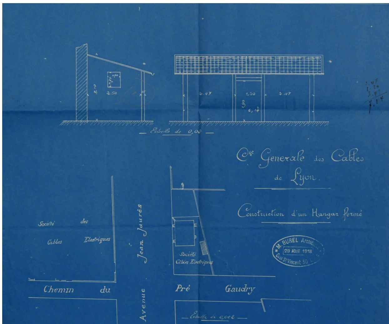
Construction d'un hangar fermé 1918 (AC Lyon 314W/603)
