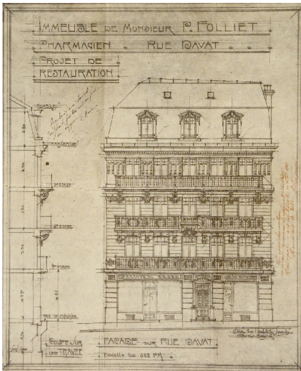
Elévation de la façade
