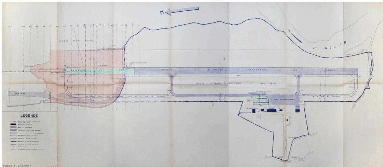
Plan d'ensemble de l'aéroport de Vichy-Charmeil, 1960, Service technique des bases aériennes (Archives municipales de Vichy).
