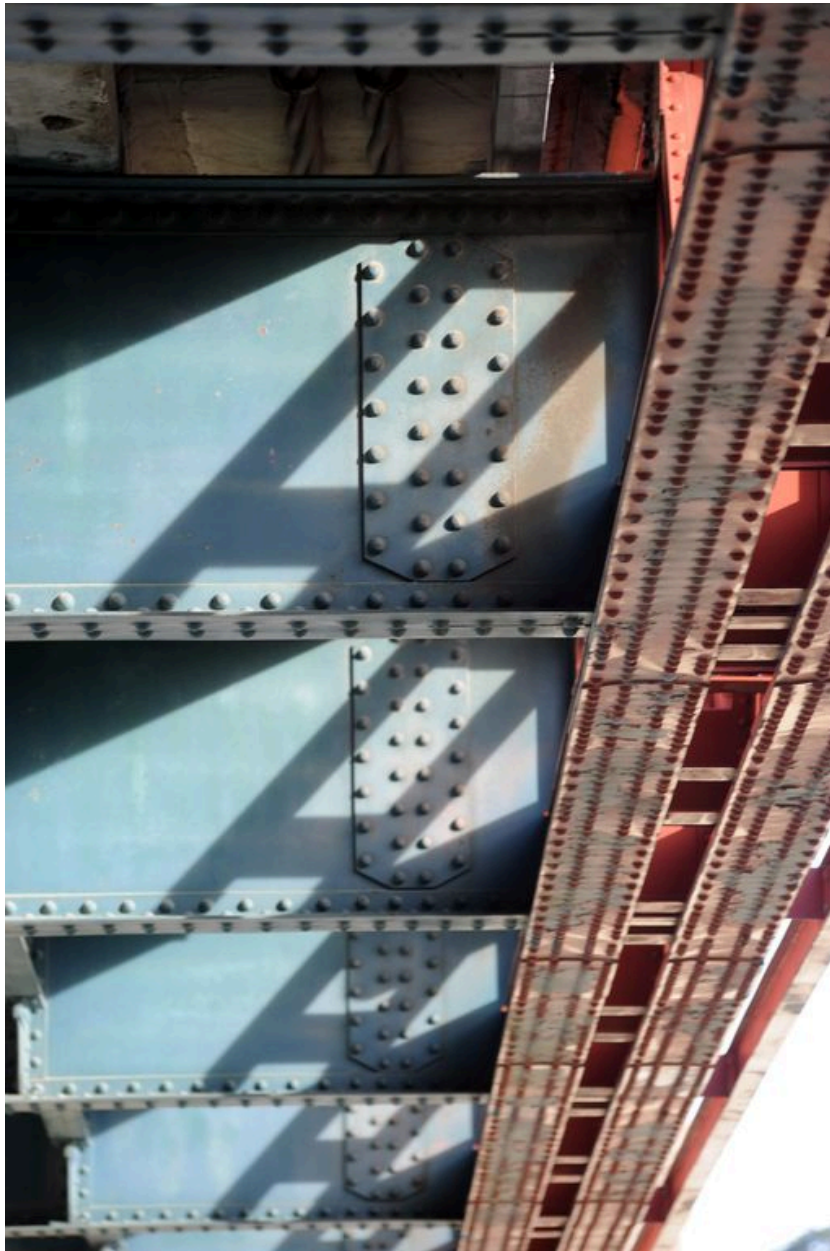
Tablier, de dessous, vue partielle : structure (depuis la rive droite)
