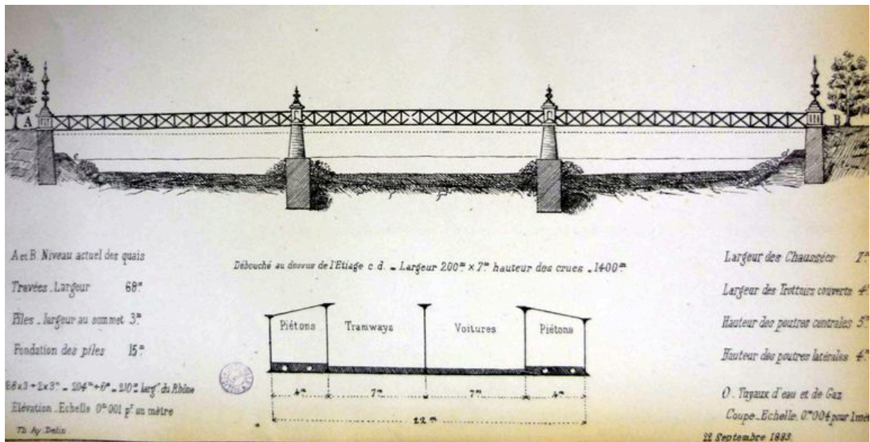
Projet d'un pont en treillis de fil de fer / Théodore Aynard, 1883
