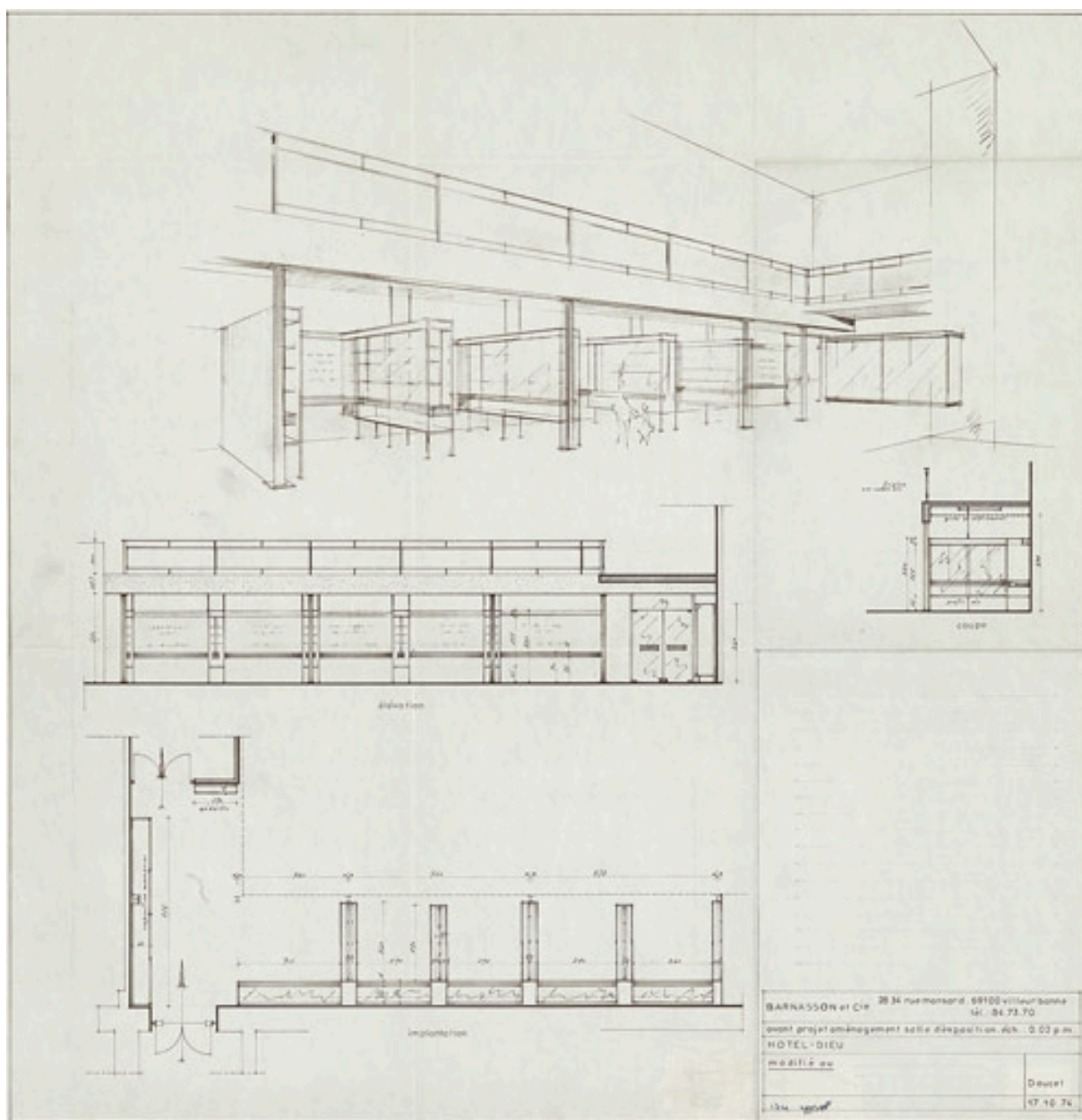
Avant-projet d'aménagement d'une salle d'exposition (Détroyat ?), plan, coupe, élévation, vue perspective, Barnasson et Cie 28-34 rue Mansard 69100 Villeurbanne, Doucet, échelle 0.02 p.m. 17 octobre 1974
