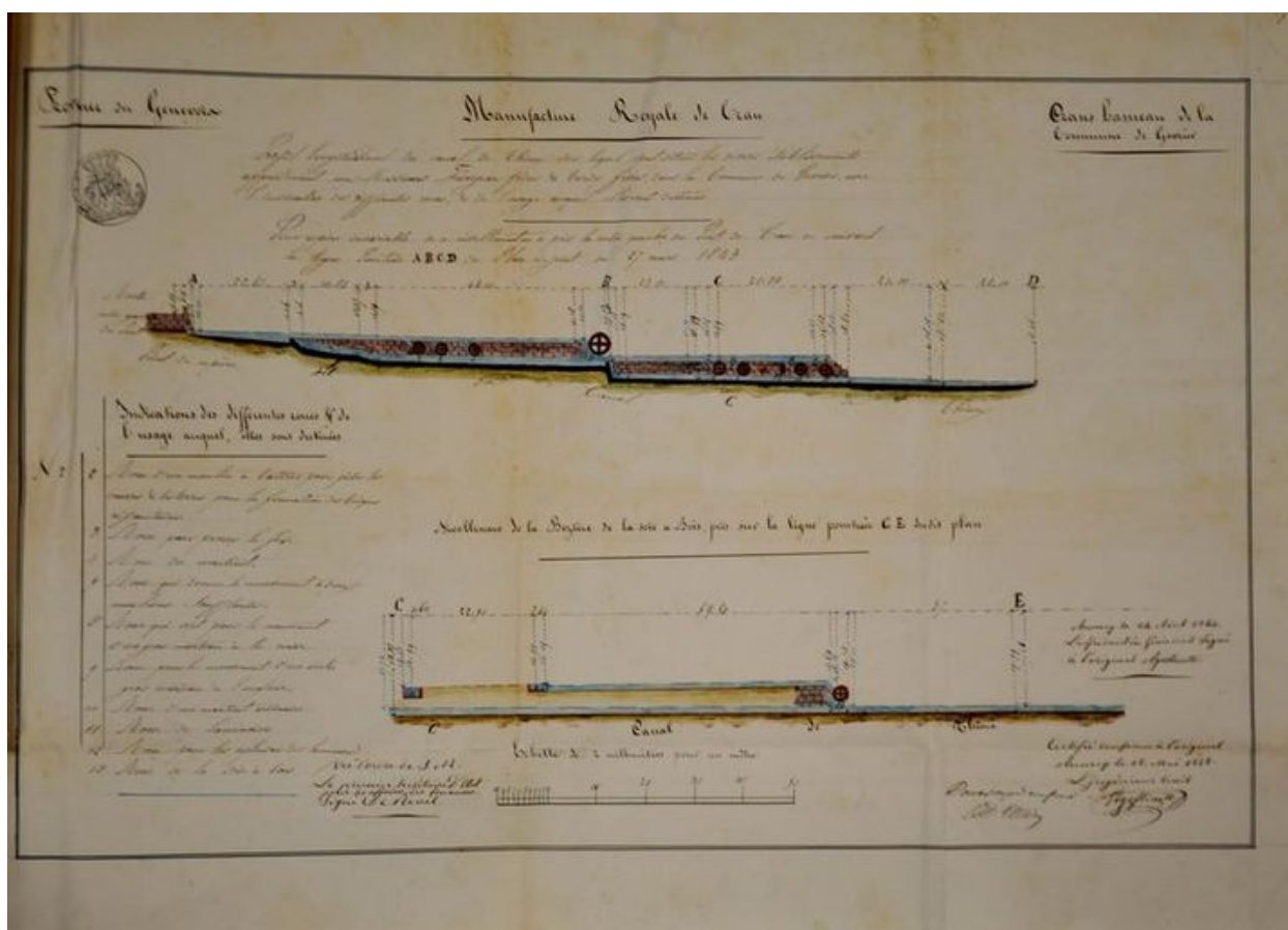
Elévation usine. Plan. Archives départementales de la Haute-Savoie © Archives départementales de la Haute-Savoie. 10 FS 45
