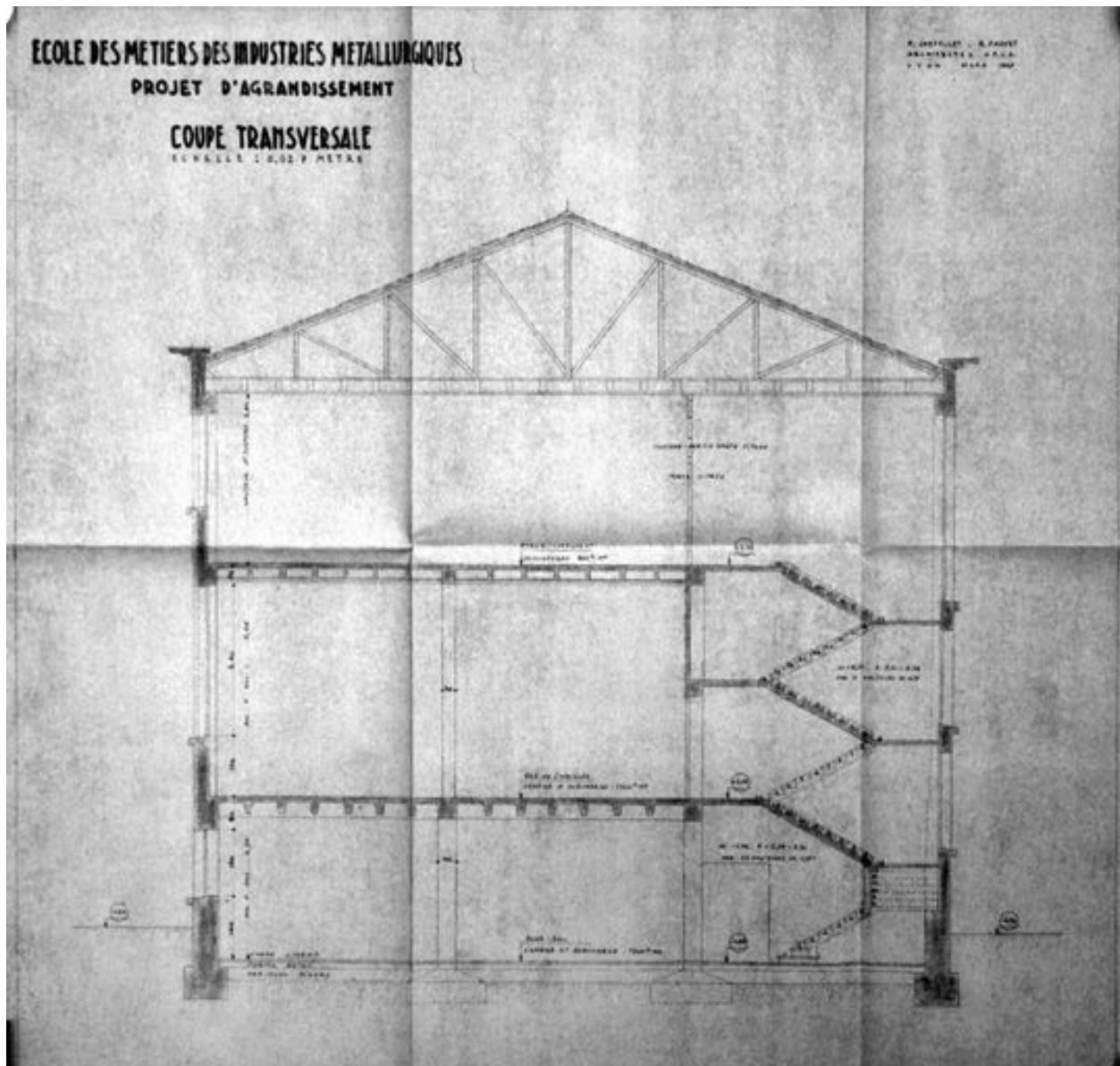
Coupe transversale (Chevallet et Fauvet), 1949
