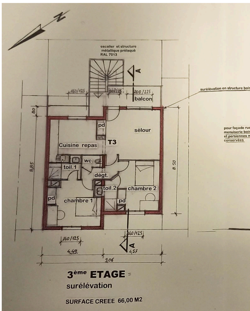
Plan du troisième étage (surélévation)
