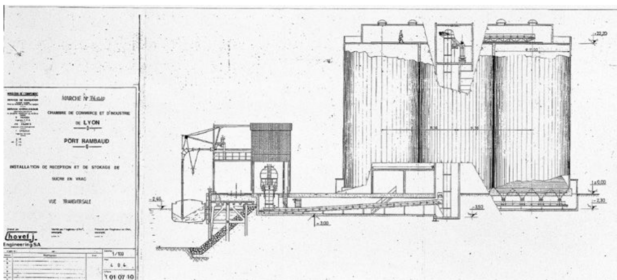
Coupe transversale sur les silos, 1975
