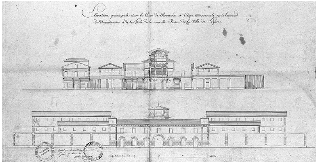
Elévation principale sur le cours de Perrache et coupe transversale sur le bâtiment de l'administration et de la geôle de la nouvelle prison de la ville de Lyon, par l'architecte Dumont, 17 mai 1827. 39 x 72,5 AD, Rhône. 1 Y 299
