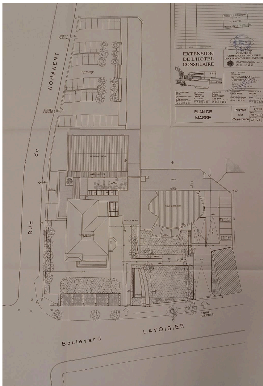
Plan masse 148 boulevard Lavoisier en 2001
