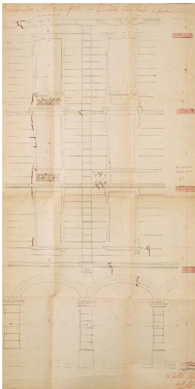
Feuille n°8. Transformation du Collège en Lycée. Elévation d'une travée de façade (1885)
