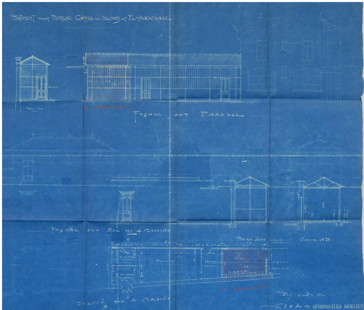
Plans 1916, bâtiments pour bureaux et embauche usine Berliet, Lyon 8e (ACL314w574-104)
