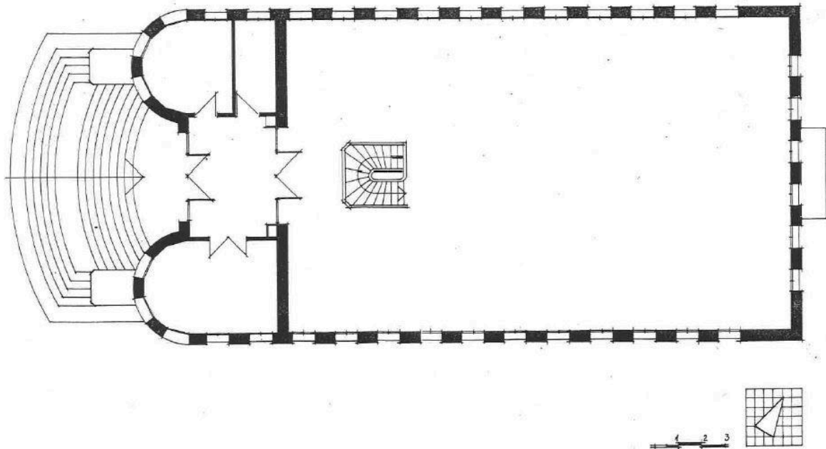
Plan du 1er étage (archive Drac Rhône-Alpes, E. Deloche, 1985)
