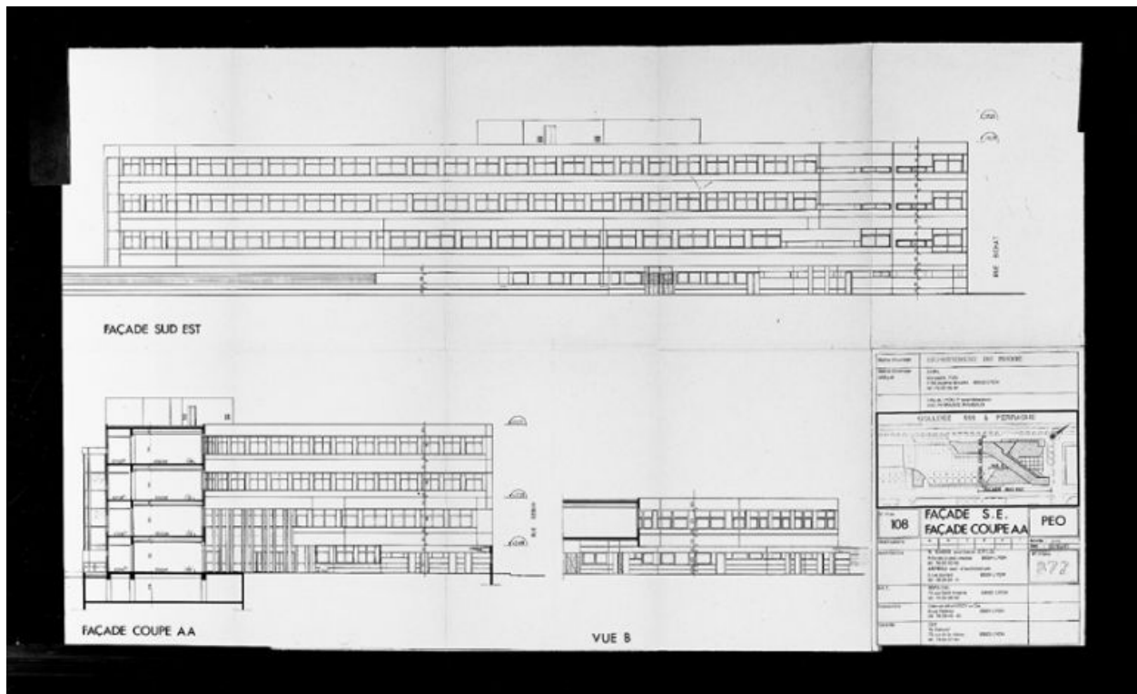
Façade et coupe AA, façade sud-est
