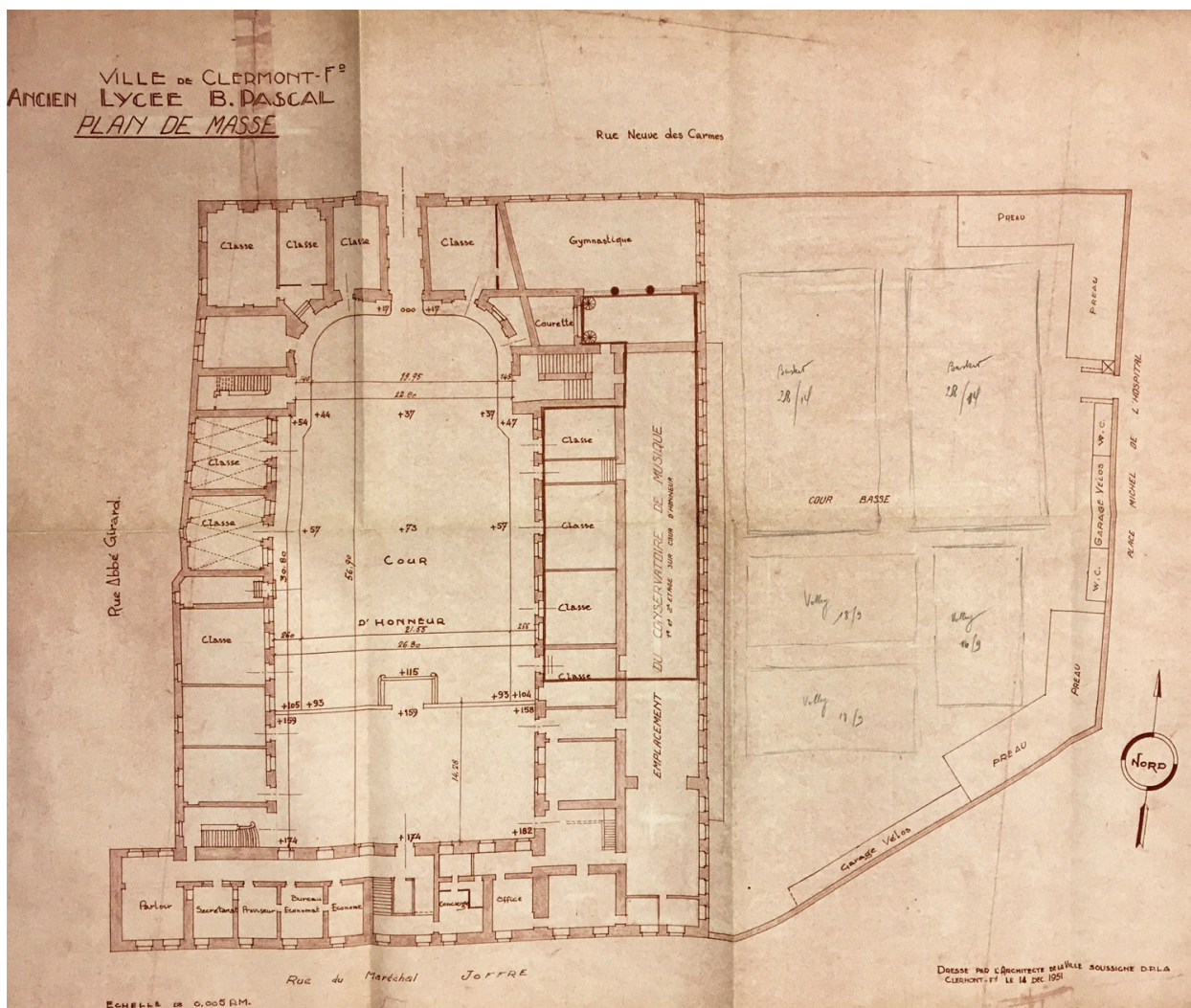
Plan masse (rez-de-chaussée) en 1951 (AC Clermont-Ferrand, 477 W 2)
