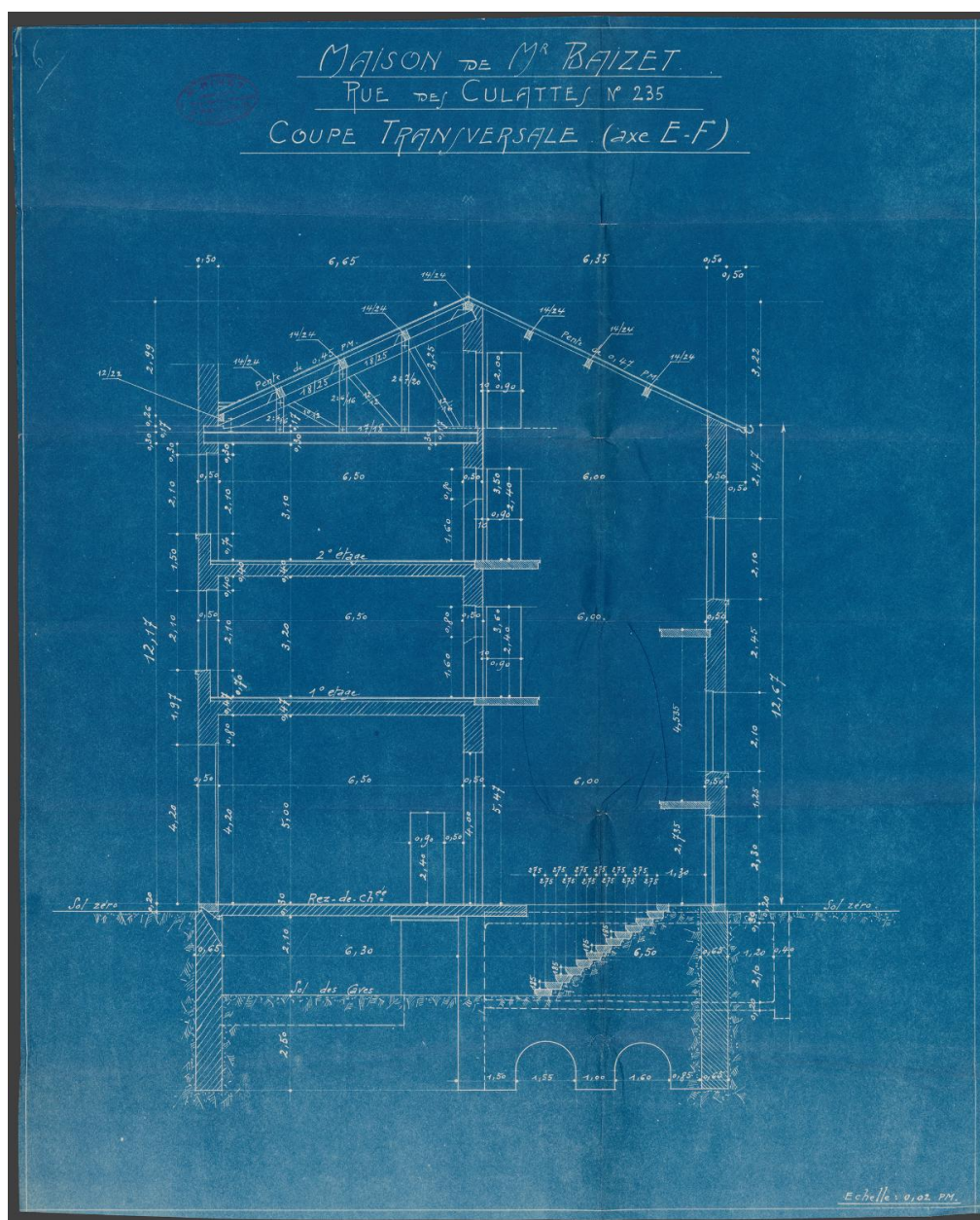
Coupe transversale, (axe E-F), P. Pinet architecte.
