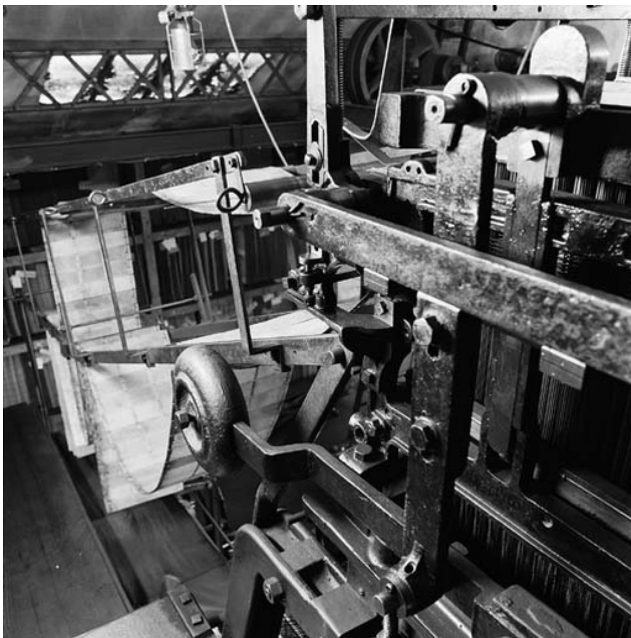
Détail mécanique du métier Biol
