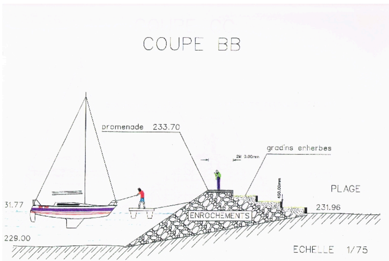
Coupe sur l'enrochement, 1991
