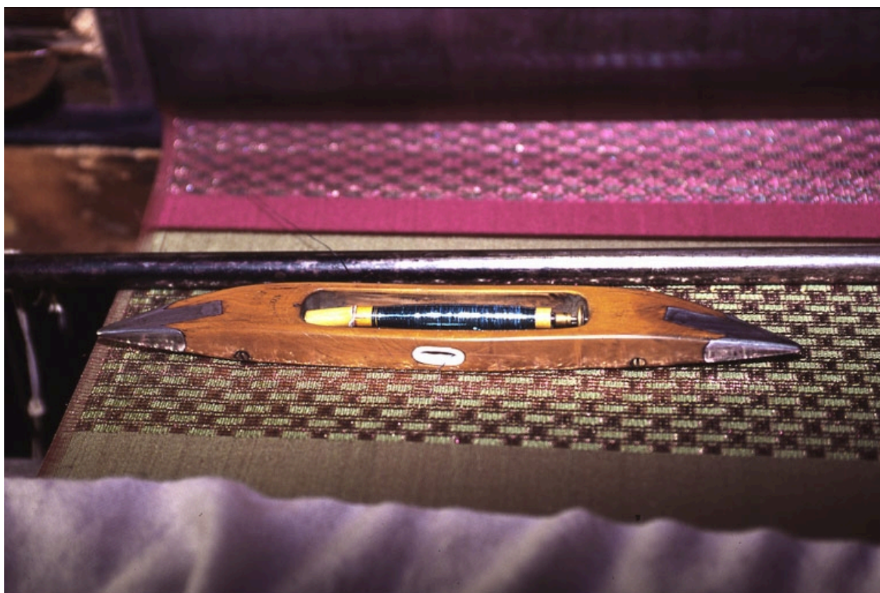
Navette à pointe-sel à rotation
