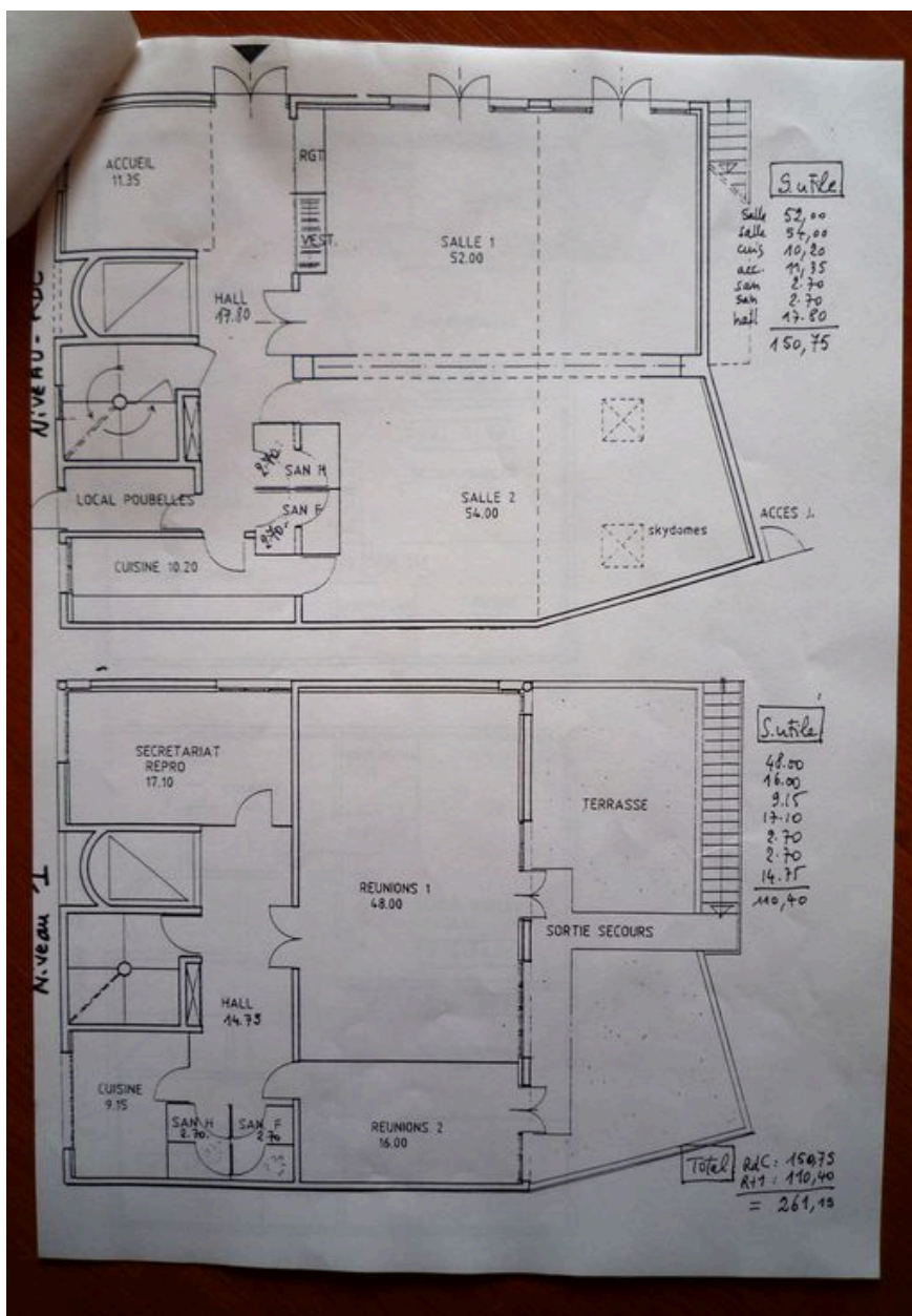
Maison paroissiale : plan du rez-de-chaussée et du premier étage
