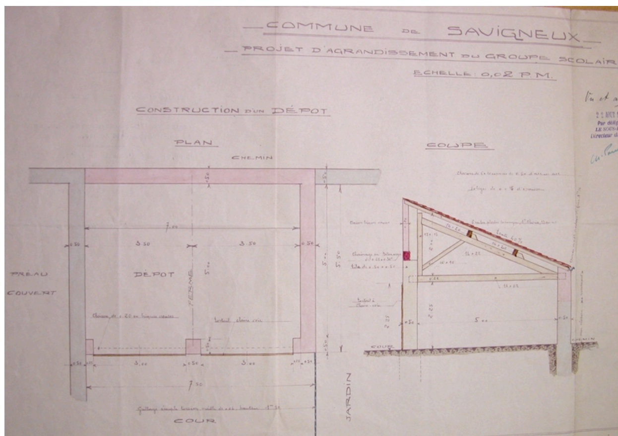
Commune de Savignieux. Projet d'agrandissement du groupe scolaire. Construction d'un dépôt. Plan. Coupe. 1928.
