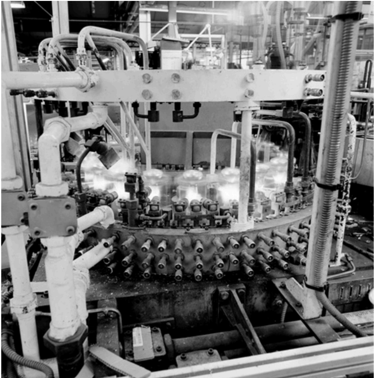
Ligne fermeture du pied de l'ampoule
