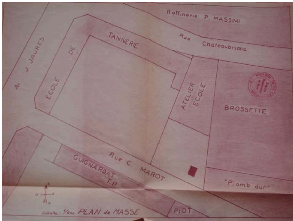
Plan du Centre Technique du Cuir ; atelier ; plan de masse
