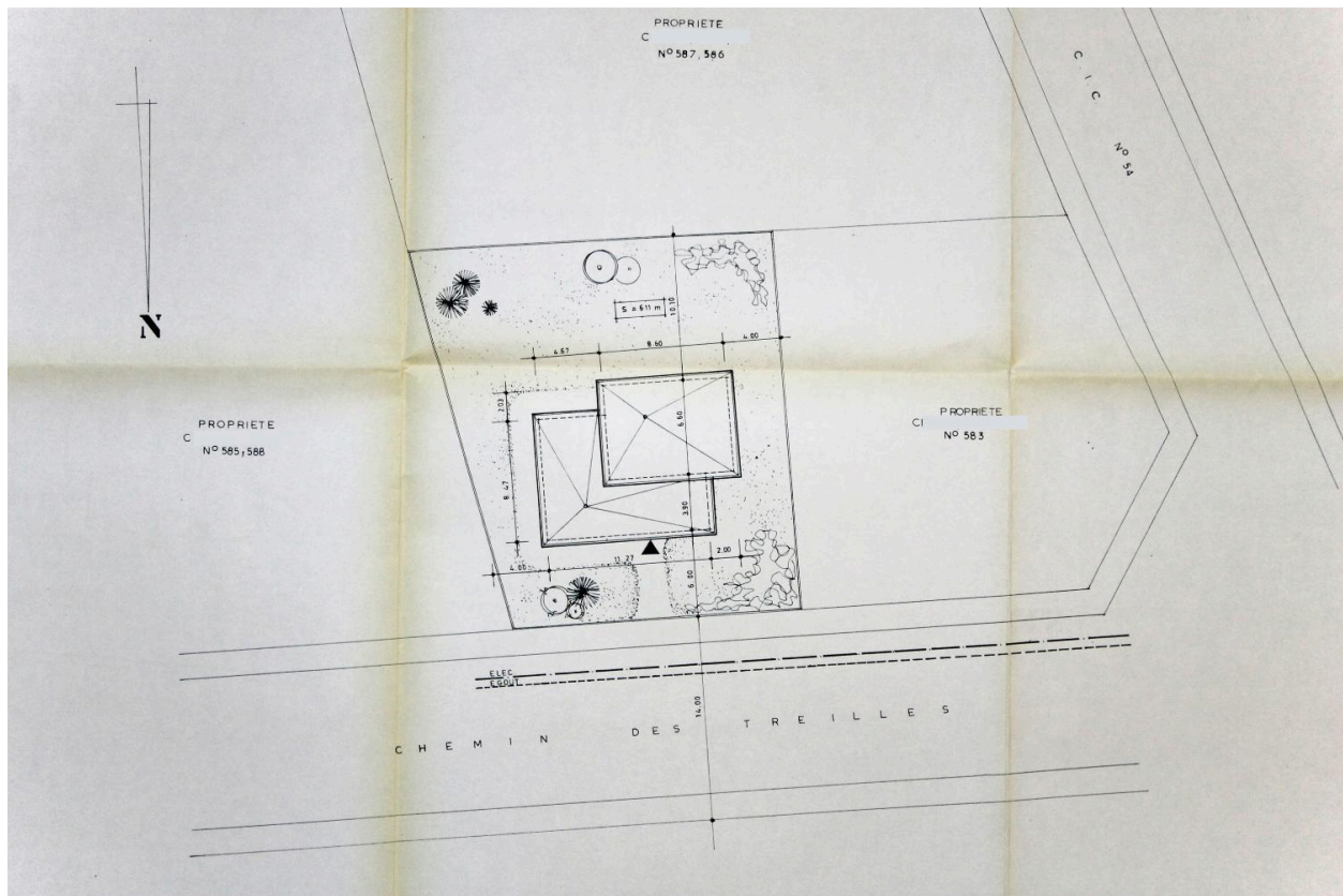
Aulnat, la Maison B.-C., plan d'implantation, 1972, Gilles GALLON architecte (Archives municipales d'Aulnat).
