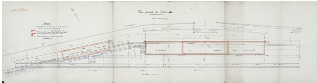
Plan général de l'estacade, projet 1913 ? (archive VNF)
