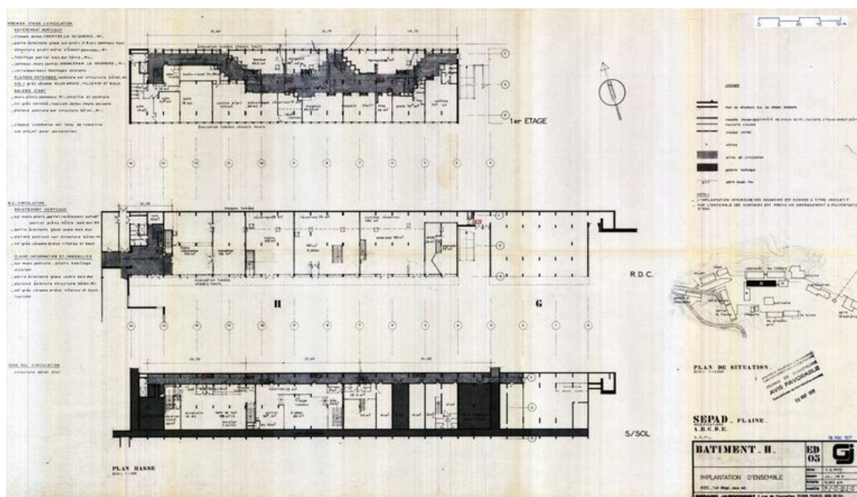
Bâtiment H. Plan de situation. Plans des sous-sol, rez-de-chaussée et 1er étage. Gérard Jardonnet architecte d'intérieur. 7 février 1977. Modifications 6 mai 1977 (AC Arâches-la-Frasse)
