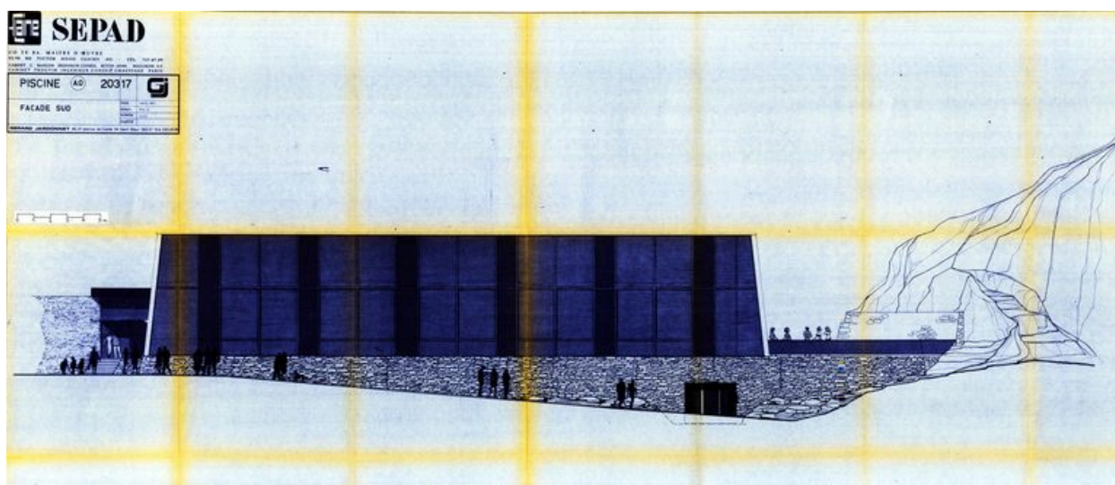
Elévation sud. Gérard Jardonnet architecte, 18 février 1971 (AC Magland)
