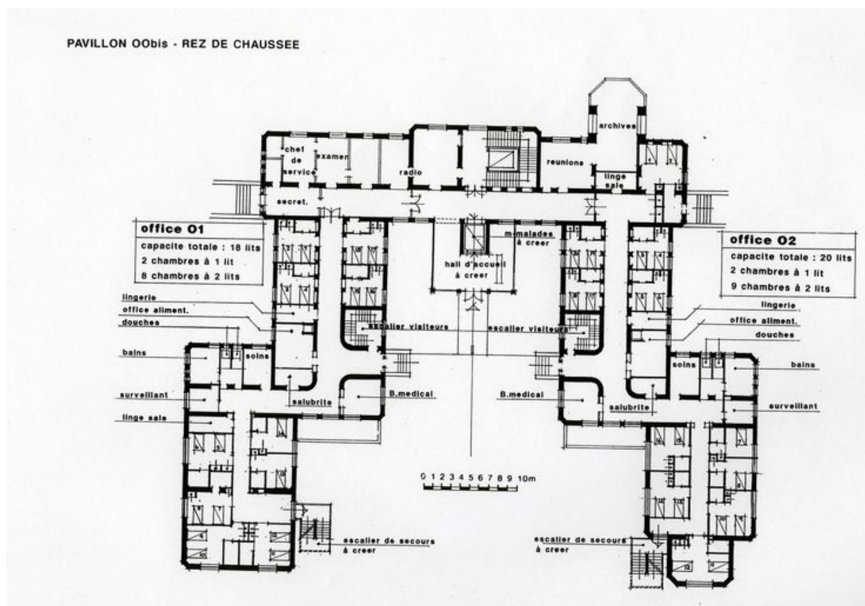
Plan du pavillon OObis. Rez-de-chaussée / E. Gachon, 1989. In : Projet d'actualisation du plan directeur
