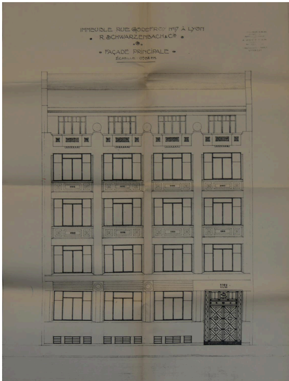
Façade principale 1929 usine Schwarzenbach (AC Lyon 344W/881 dossier 1045)
