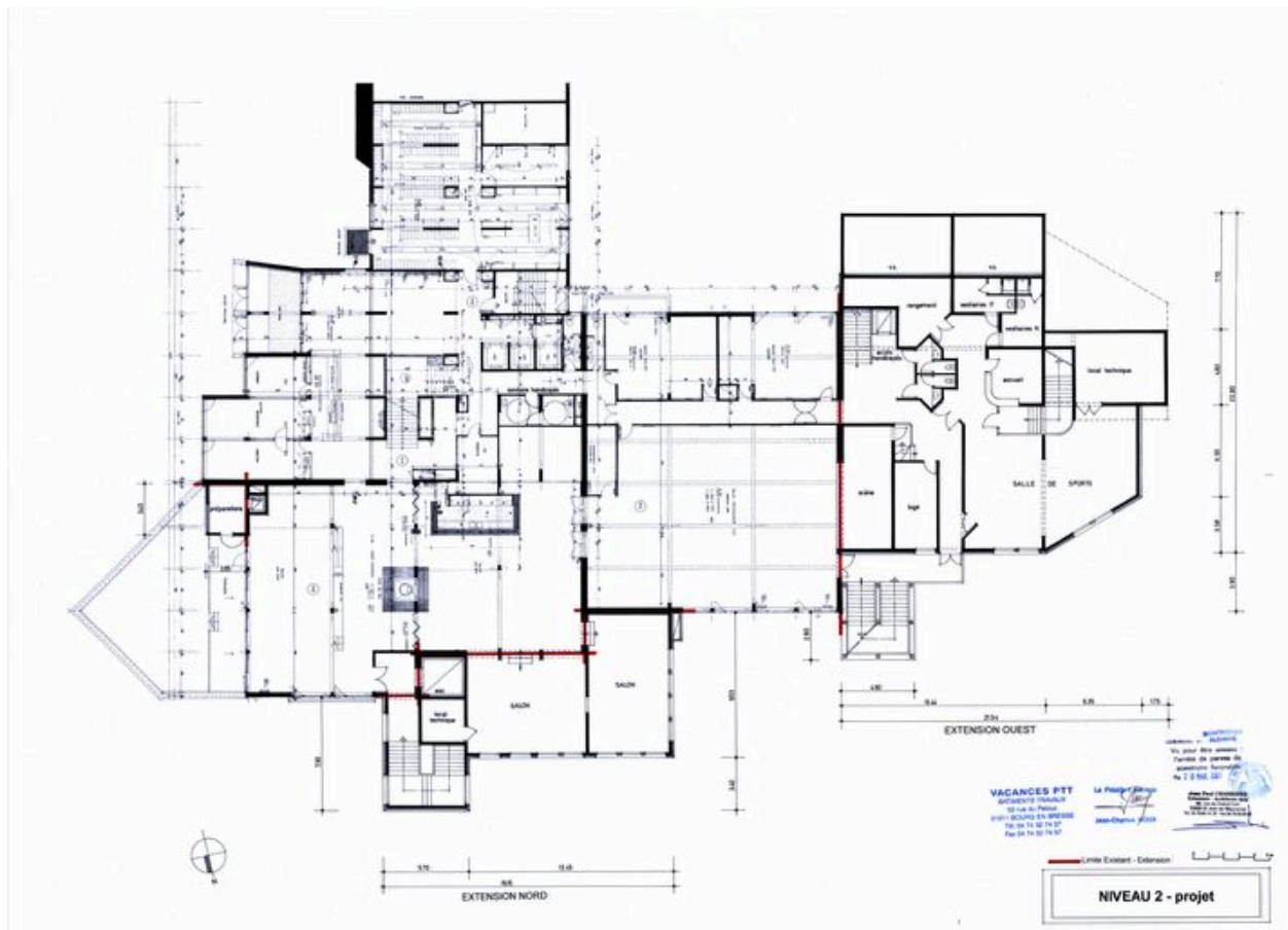
Centre de vacances Azurèva. Projet de requalification et d'agrandissement des parties communes. Plan du niveau 2 / Jean-Paul Charrière, 2000 (AC Montricher-Albanne)
