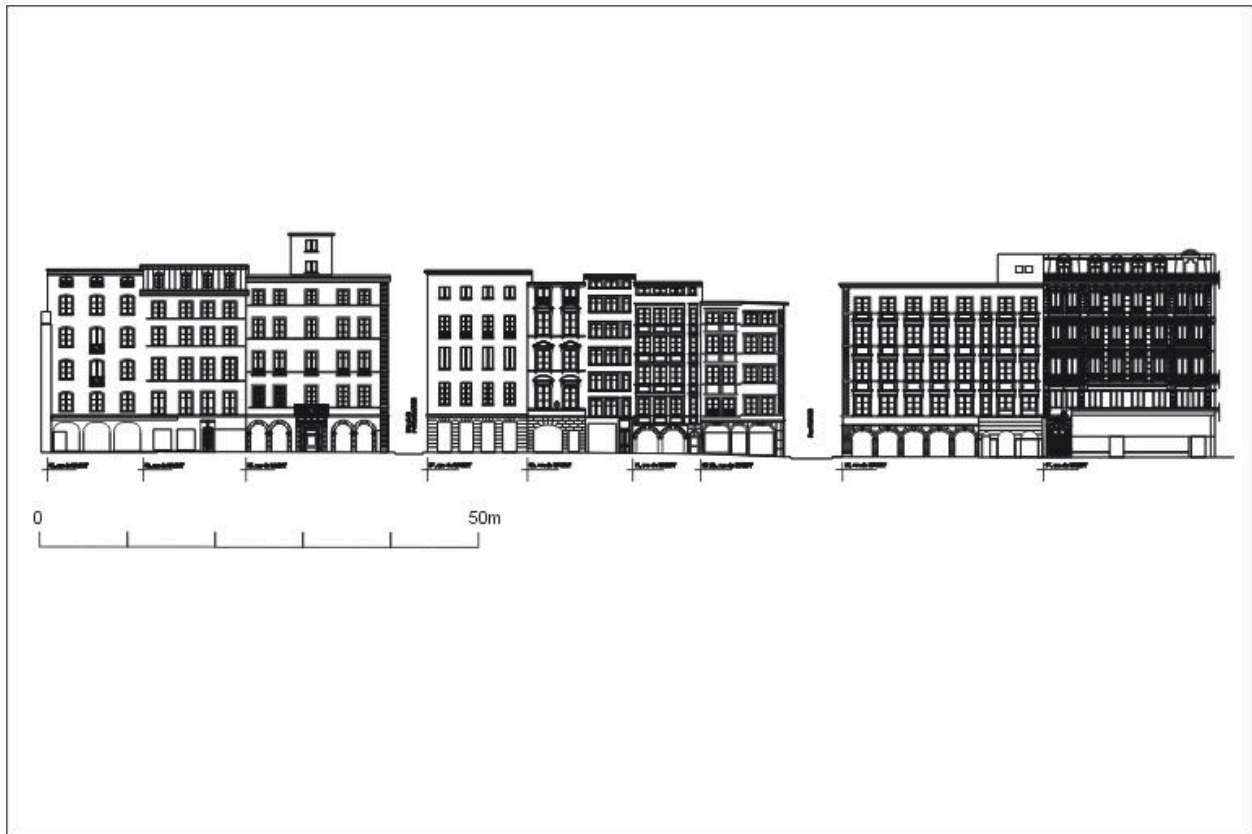
Elévation du côté est de la rue de Brest, entre l'église Saint-Nizier et la rue Grenette, d'après un relevé photogrammétrique par A. Bensaci, 2003
