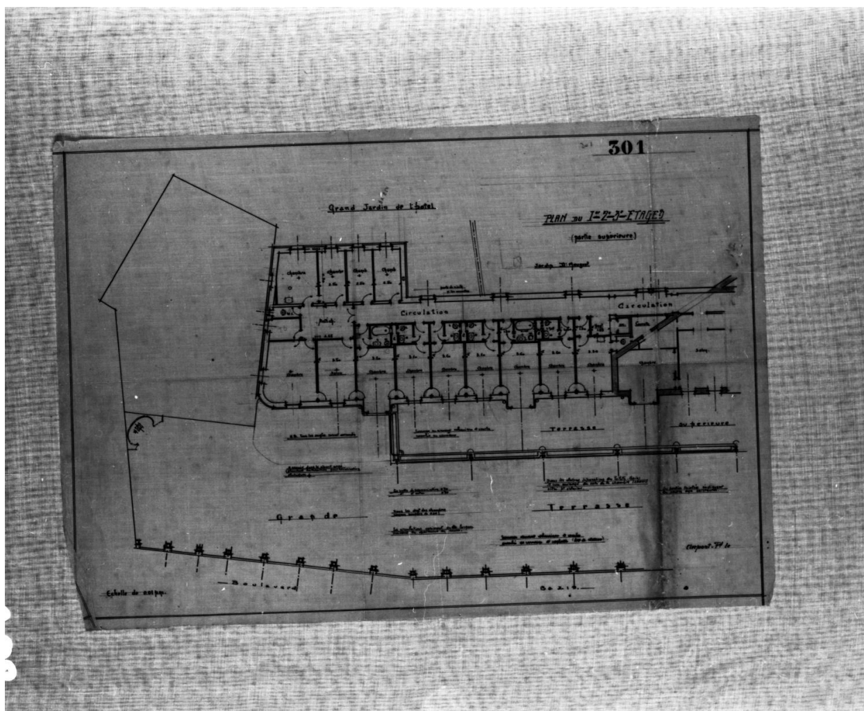
Plan des premier, deuxième et troisième étage du Royat-Palace vers 1920
