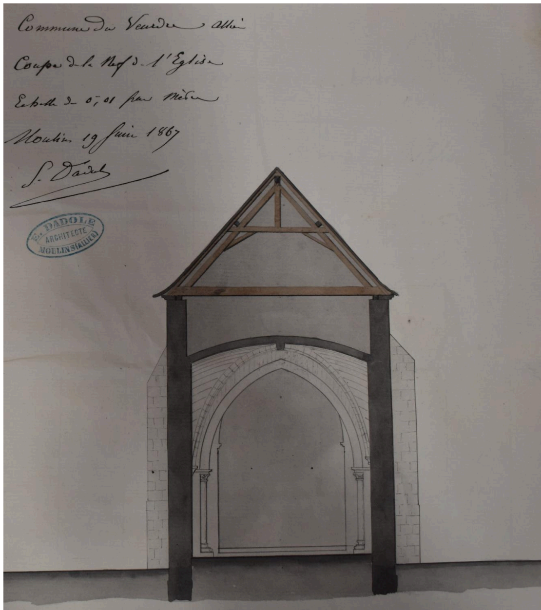
Coupe de la nef de l'église par Emile Dadole, Moulins, 1867.
