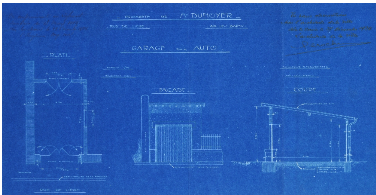
Plan, coupe et élévation du garage
