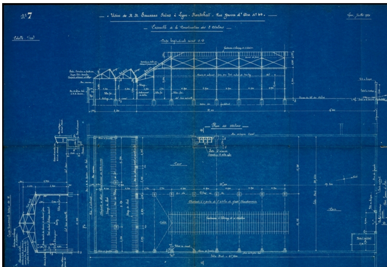
Plan et coupe de l'usine pour messieurs Sassac frères, 1920. AC Lyon : 324 WP 062 PCA n°502
