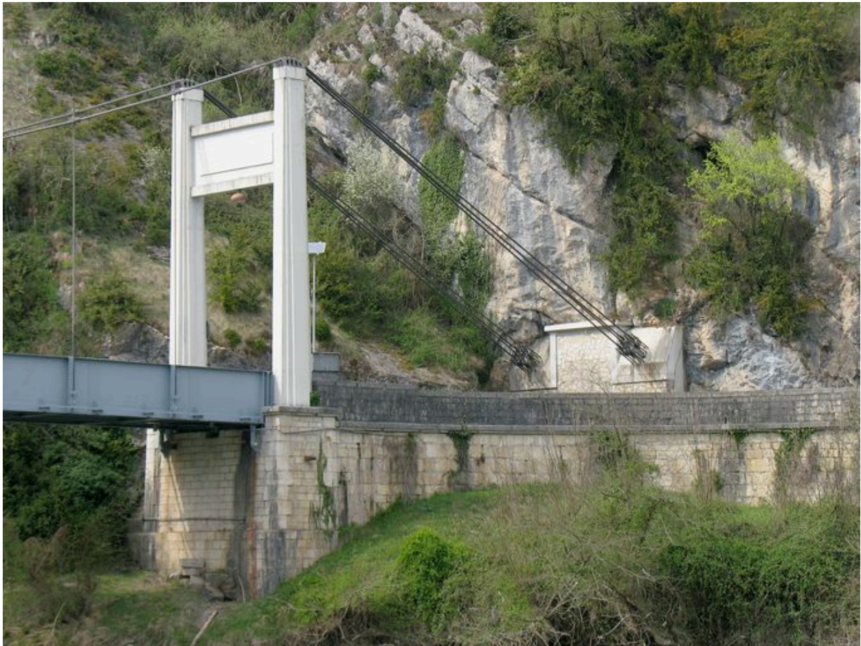
Vue partielle, pylône et culée droits, face amont (depuis la rive gauche)
