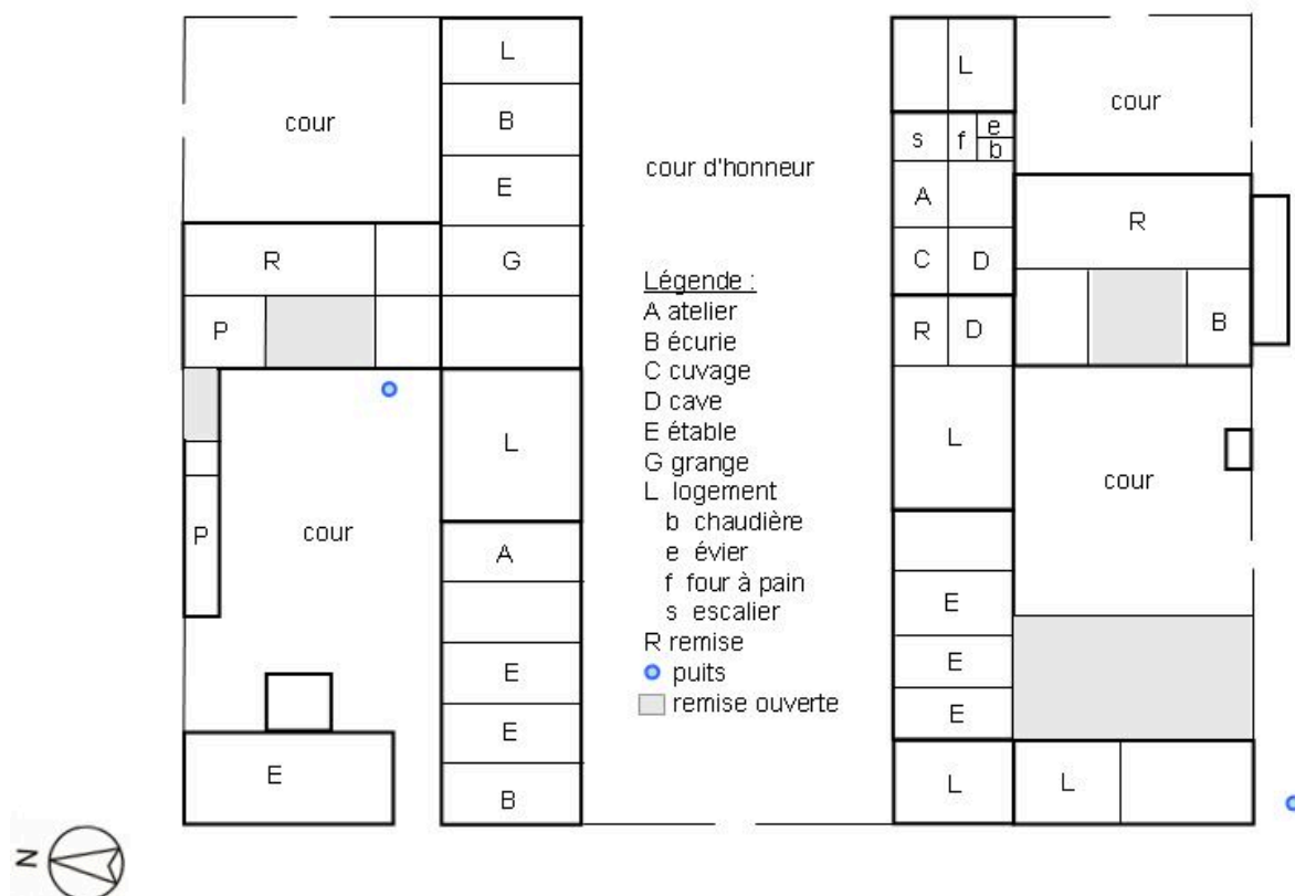
Plan-masse.
