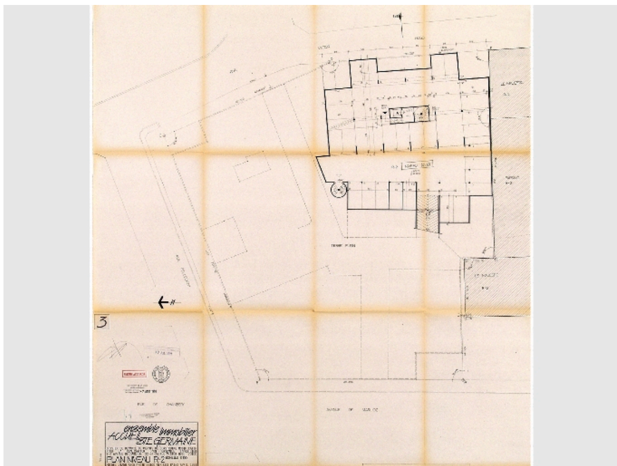
Plan du 2e sous-sol
