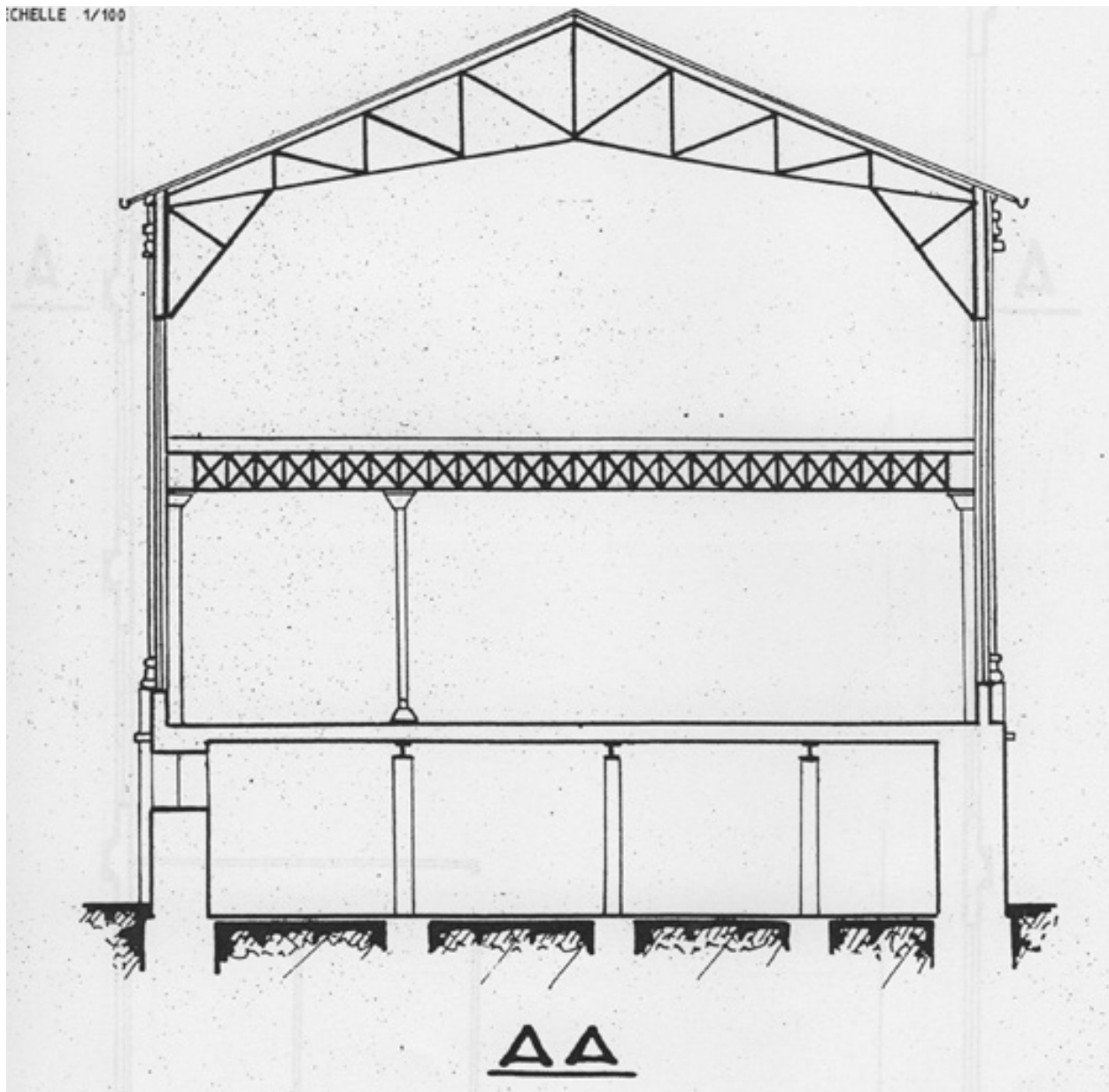
Coupe AA : dressé par le cabinet Lecart, janvier 1942
